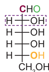
D-Allose
