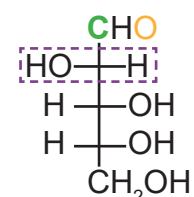
D-Arabinose
