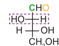
D-Threose
