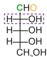
D-Ribose
