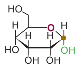
\alpha -D-Allose
