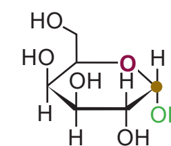
\alpha -D-Galactose
