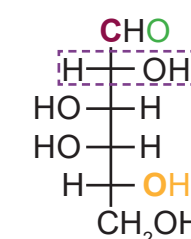
D-Galactose
