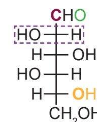
D-Idose
