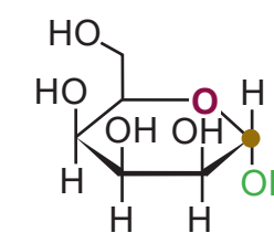
\alpha -D-Talose
