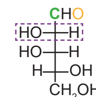
D-Lyxose
