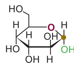
\alpha -D-Altrose
