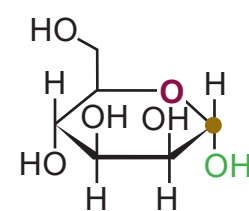
\alpha -D-Mannose
