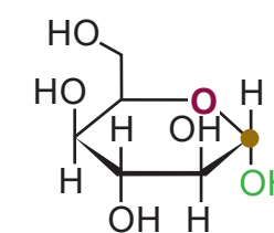
\alpha -D-Idose
