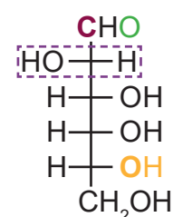
D-Altrose
