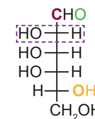
D-Talose
