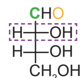
D-Erythrose
